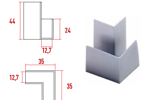
D228 Sunta Kenar Koruma Plastiği
