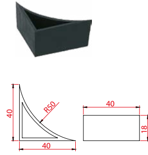
P8008 Pressia Köşe Plastiği
