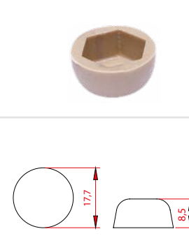
D122 Şapkalı Klapa Dübeli
