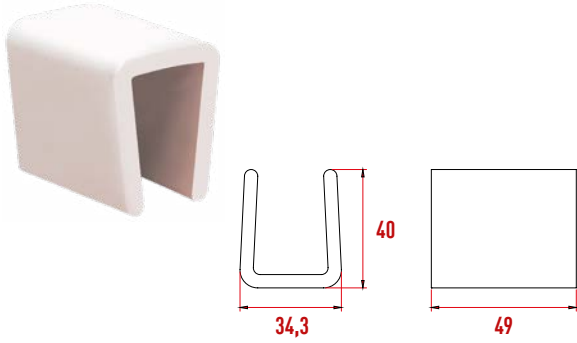
P2014 N Maşa
