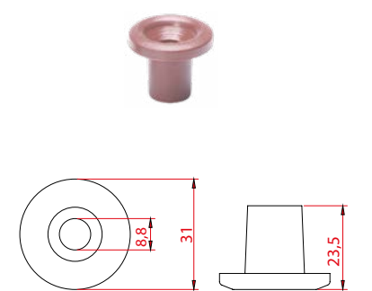
P1207 Kasa Koruyucu Delikli Tıpa
