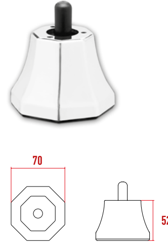
P987 Verona Ayak Krom Çakmalı
