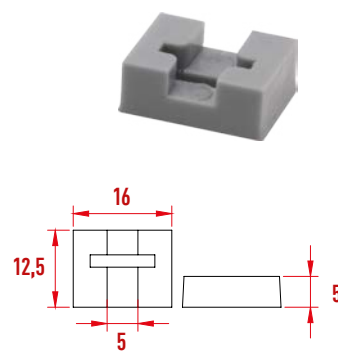
P3105 27'lik Stoplama Plastiği
