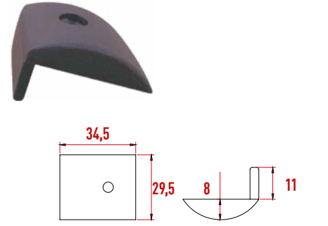
D124 Baza Denge Takoğu 8 mm
