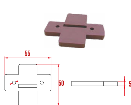
P3064 Menteşe Yükseltici 5 mm
