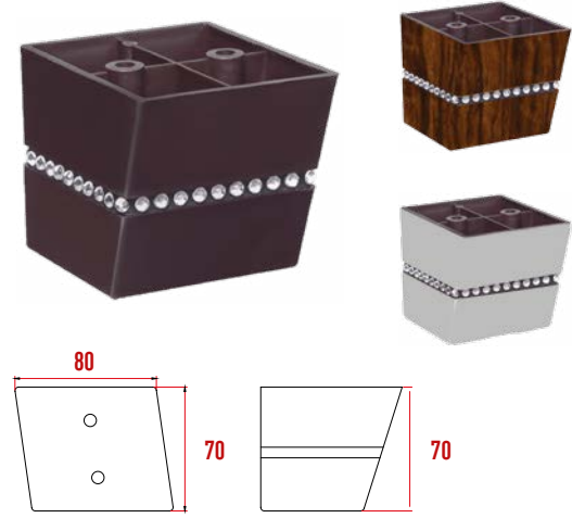
P908 Karizma Berjer Ayak
