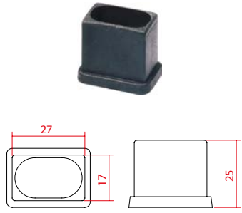
P1500 Yeni Delikli Takoz
