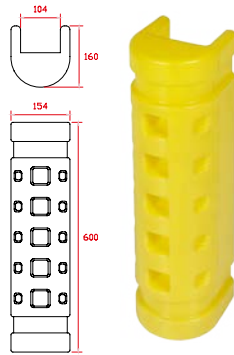
D297 Raf Koruma Plastiği
