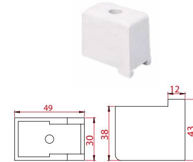
D162 Royal Ray Takozu
