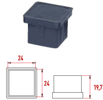
D119 Profil Takozu 25x25 mm
