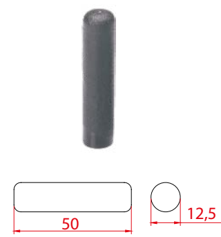
P1510 Ahşap Ayak Pimi
