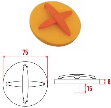
P3080 Soldier Kulp
