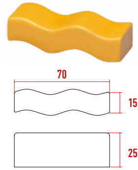
P3003 Slide Kulp
