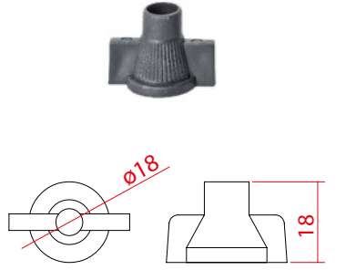
D177 Kelebek Somun M6
