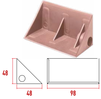
P1102 Kısa Orta Köşebent 98 mm
