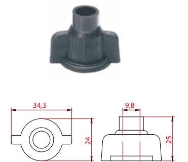
D176 Kelebek Somun M8
