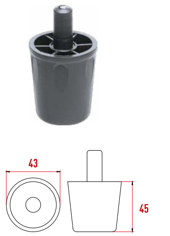
P949 Gizli Ayak Çakmalı 45 mm
