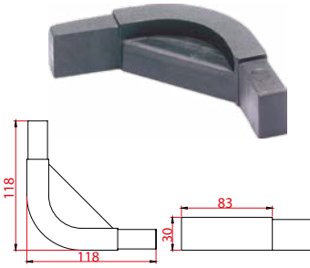
P2018 Profil Köşe Geçme 20x30
