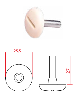
P1512 M6 Konik Bağlantı Vidası
