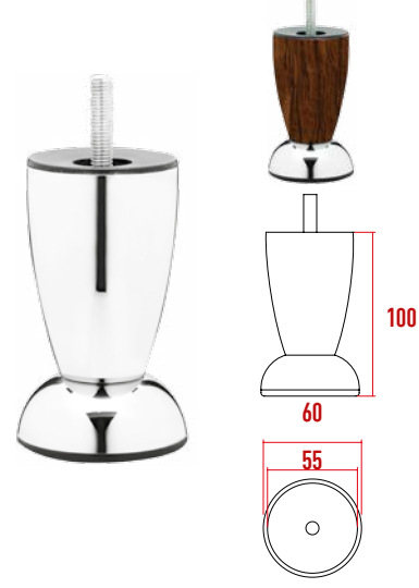
D235 Milano Ayak 100mm
