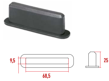
P2012 Lata Yatağı
