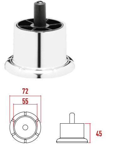
P982 Kelepir Ayak Çakmalı 45 mm
