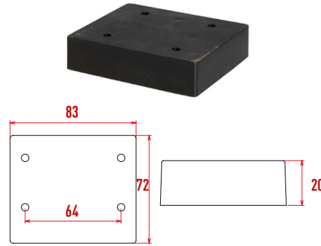
P3142 Hanzade Yükseltici
