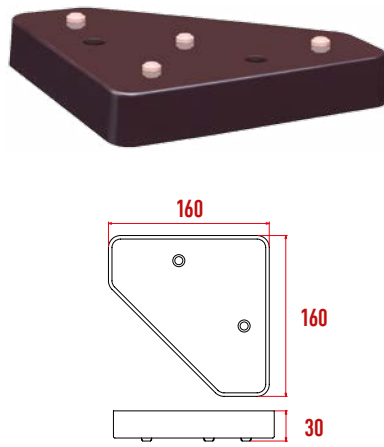
P1023 Premium Ayak
