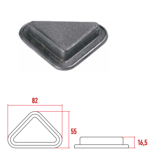
P1058 Üçgen Ayak
