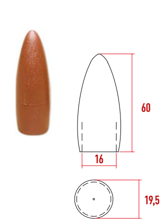
P1083 Woody Zigon Sehpa Ayağı 16'lik
