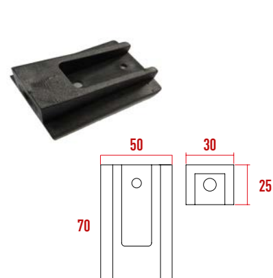
Y404 Gizli Ayak Bağlantı Pls. Kulaklı
