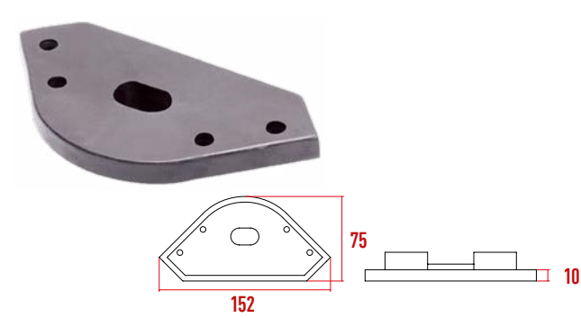
P2024 Stop Silindiri
