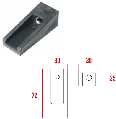
P1105-1 Gizli Ayak Bağlantı Pls. Merit Pimli
