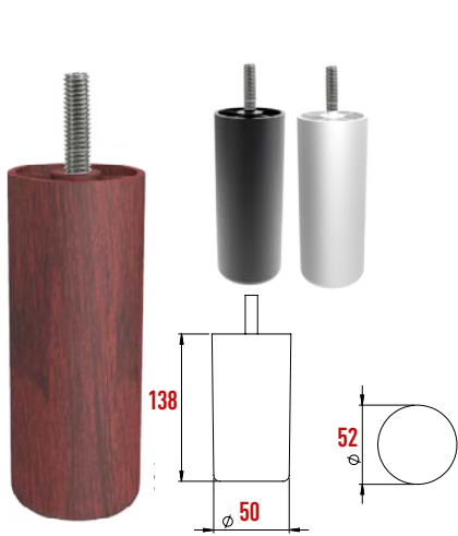
V316 Gizli Ayak 138 mm
