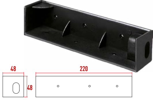
P1118 Takviyeli Köşebent 222 mm
