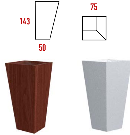
P1705 Domino Berjer Ayak 143 mm
