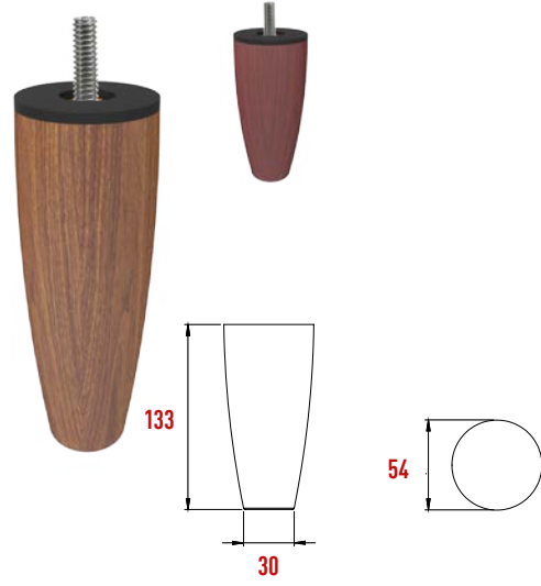
V306-133 Gizli Ayak 133 mm
