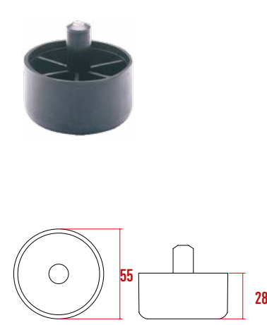
P1015 Galaxy Ayak Geniş
