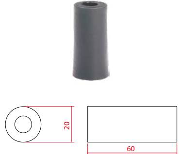
P1410 Kol Ara Bağlantı Silindiri 60 mm
