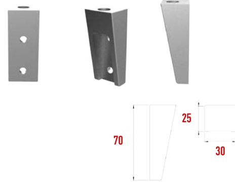
P1105-5 Gizli Ayak Bağlantı Pls. Çakmalı
