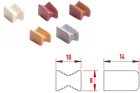
P3010 Kırılmaç Kama 14 mm
