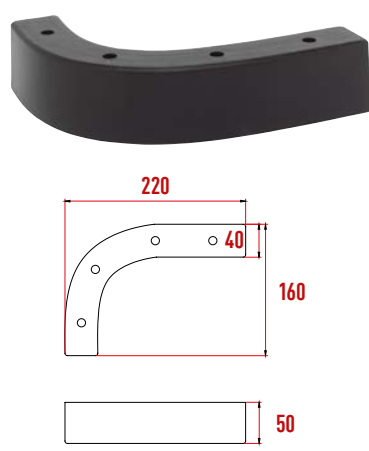
P3125 Prestij Ön Ayak
