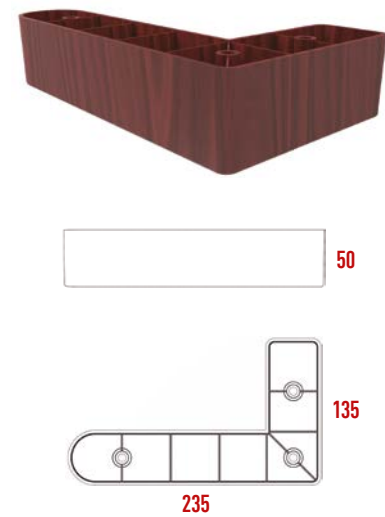
R290 Tunus Ayak
