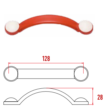
P3019 Sunlight Kulp
