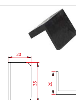
P1305-2 Boytaş Pvc L Siyah
