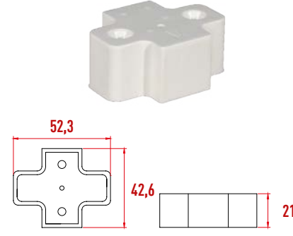
P3032 Kitaplık Ray Yükselticisi 21 mm
