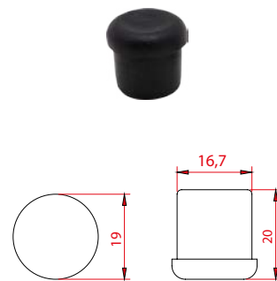
D129 Boru Takozu 19'luk
