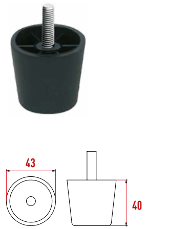
P906 Gizli Ayak Cıvatalı 40 mm
