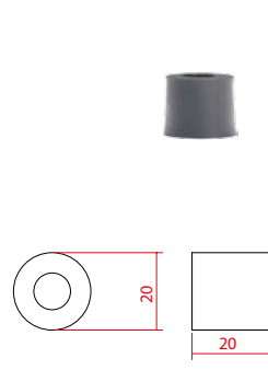
P2023 Kol Ara Bağlantı Silindiri 20 mm
