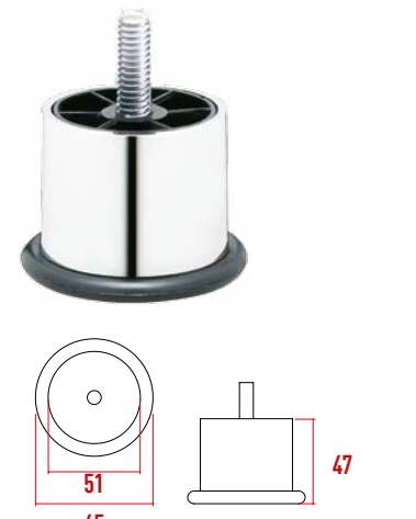
P1035 Metal Ayak
