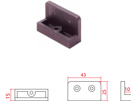
P1408 Royal Ray Stobu
