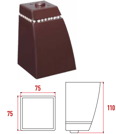
P923 Retro Berjer Ayak Metal Şeritli
