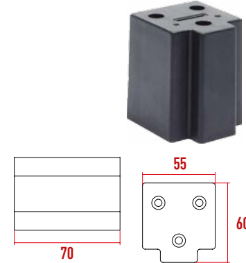
P3081 Rio Menteşe Yükseltici 70 mm
