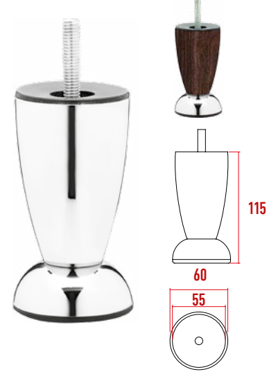
D295 Milano Ayak 115mm
