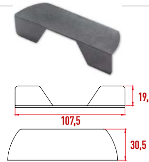
P1204 Yatak Köşe Koruyucu
