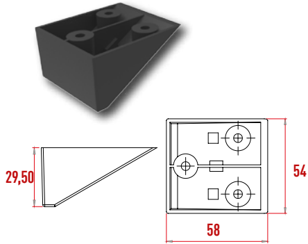
R269 Açılı Menteşe Yükseltici
