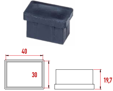
D146 Profil Takozu 30x40 mm
