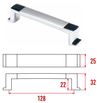
P3092 Melodi Kulp
