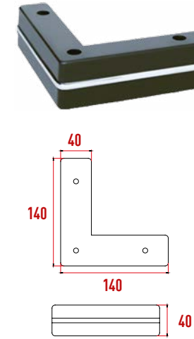
P934 Karel Köşe Ayak
