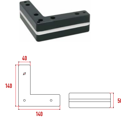
P929 Dream Köşe Ayak
