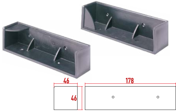
P1103 Takviyeli Köşebent Kısa
