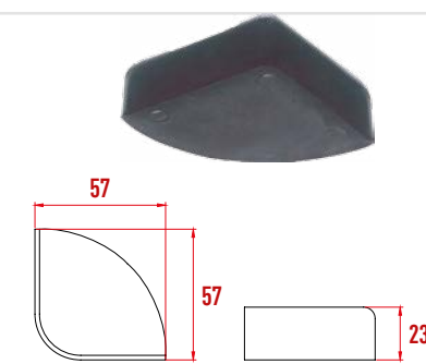
P1200 Alt Kasa Kanep Koruyucu
