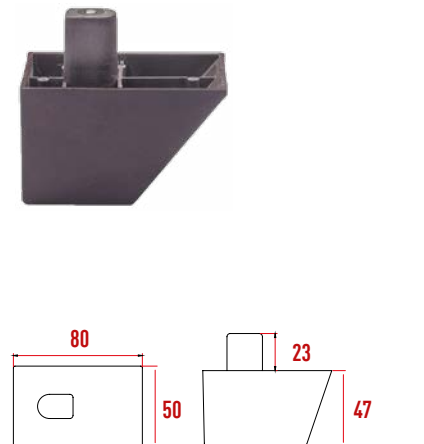
P1004 Remo Ayak
