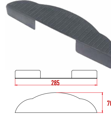
P2009 Baza Köşe Koruyucu Büyük
