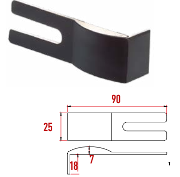
D271 Baza Dengeleme Plastiği
