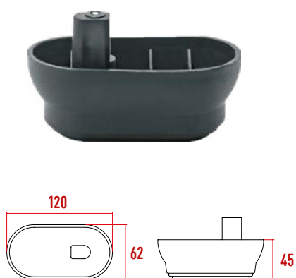
P1013 Elips Ayak
