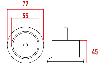
D296 Zümrüt Kol Plastiği
