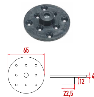
P3051 Liparis Ayak Montaj Aparatı
