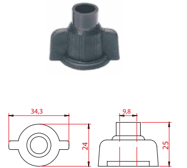
D132 Kelebek Somun 5/16
