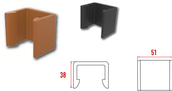
R279 Baza Birleştirici 40'lık
