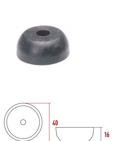
P1507 Ayak H102
