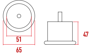
P1087 Merkür Ayak
