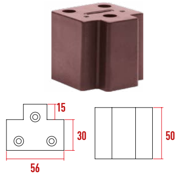
R269 Açılı Menteşe Yükseltici
