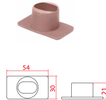
D157 Boru Takozu 38 mm
