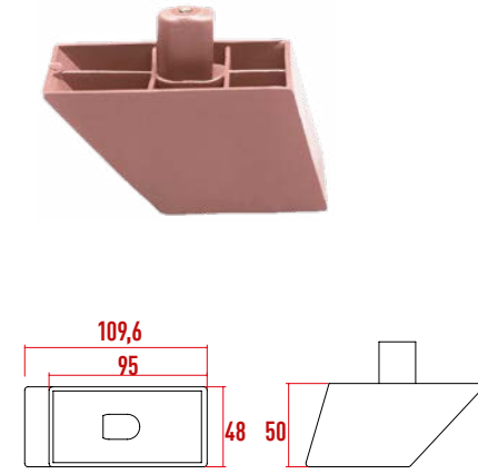
P1063 Bravo Kenarlı Ayak
