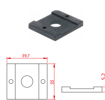
D180 Tablalı Somun Sabitleme Pls.
