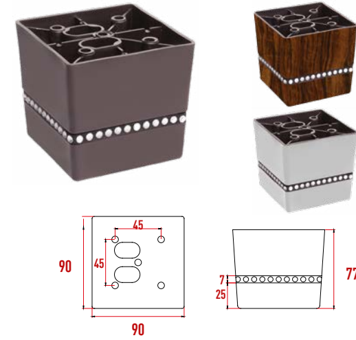
P956 Cosmo Berjer Ayak 2 No Taşlı
