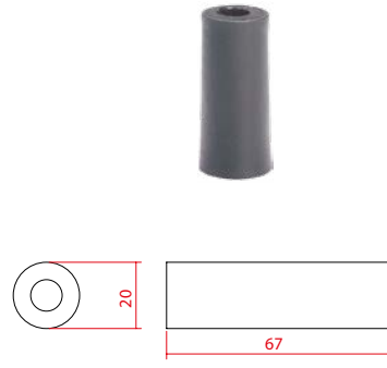
P1401 Kol Ara Bağlantı Silindiri 67 mm
