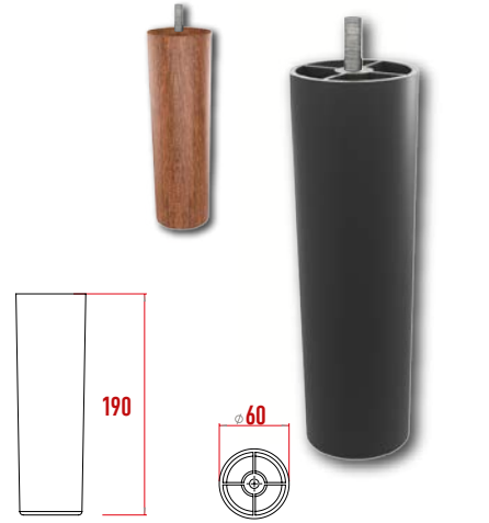
R257 Arizo Ayak 190 mm
