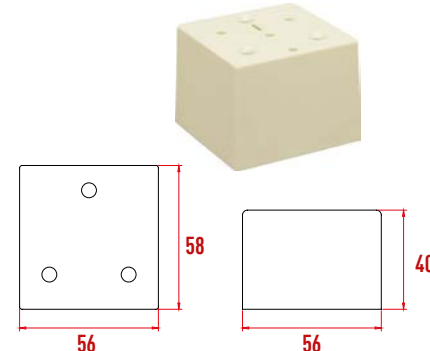
P3085 Casalisa Menteşe Yükseltici
