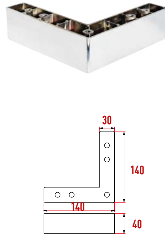
P940 Akuamarin Köşe Ayak
