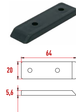
P3098 Alt Ara Bağlantı Plastiği
