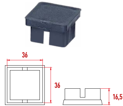
D145 Profil Takozu 40x40 mm
