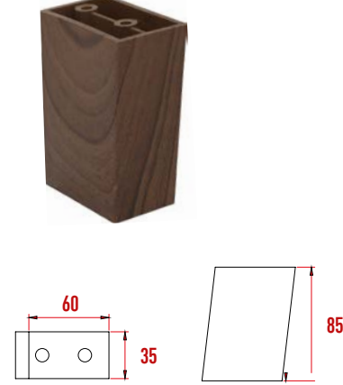
P872 Şölen Ayak Tekli
