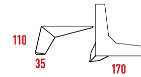
R232 Star Köşe Ayak 170 mm
