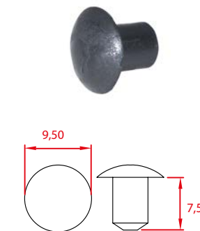
P2002 10'luk Tıpa
