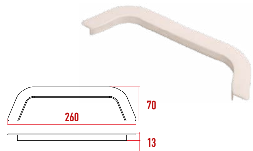
P2028 Baza Kulp Koruyucu
