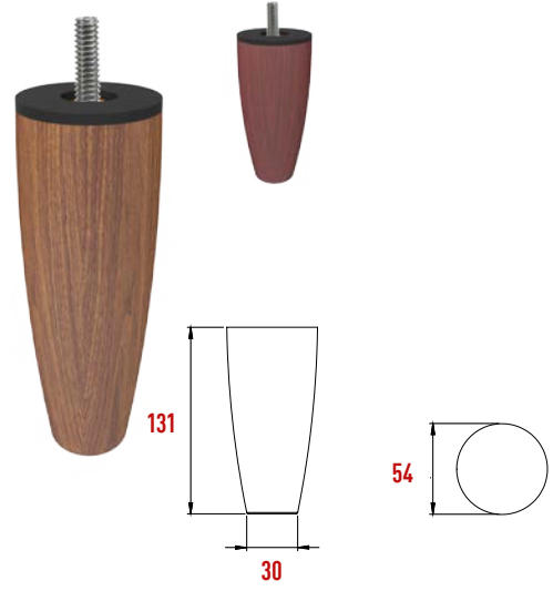
V306 Gizli Ayak 131 mm
