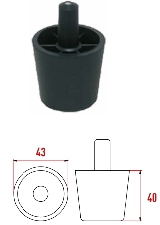
P938 Gizli Ayak Çakmalı 40 mm
