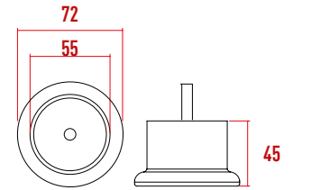
P870 Lavin Kol Plastiği
