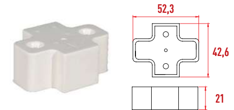
P3032 Kitaplık Ray Yükselticisi 21 mm
