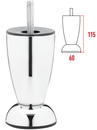
D295 Milano Ayak 115 mm
