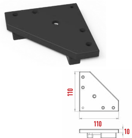
P1109-1 Üçgen Köşebent Somunlu
