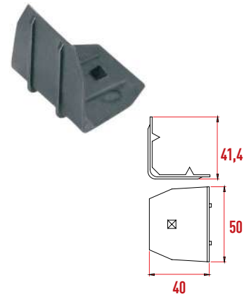
P1201 Koli Koruyucu
