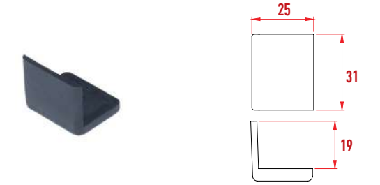
P1305 Pvc L Kahve
