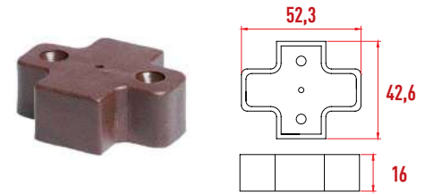
P3033 Kitaplık Ray Yükselticisi 16 mm
