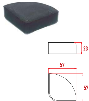
P1203 Üst Köşe Koruyucu
