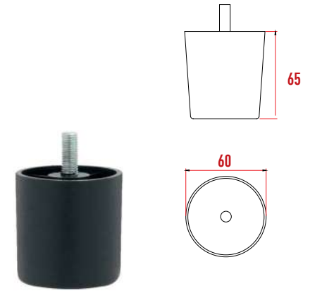
P914 Atena Gizli Ayak 65 mm
