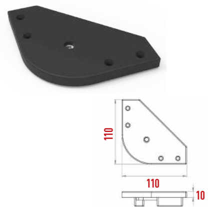
P1109-1 Üçgen Köşebent Somunlu
