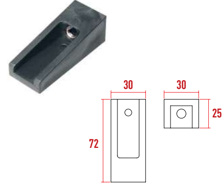
P1105-1 Gizli Ayak Bağlantı Pls. Merit Pimli
