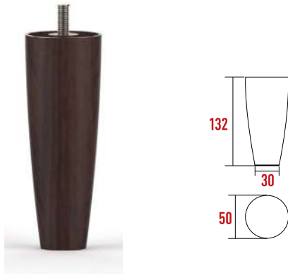
V306 Nevada Gizli Ayak 132 mm
