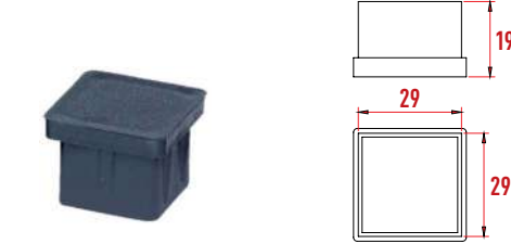
D120 Profil Takoza 30x30 mm
