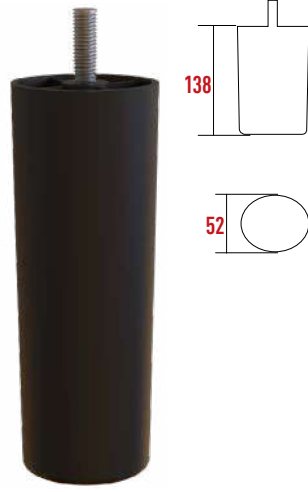
Y861 Ayarlı Ayak 95 - 138 mm
