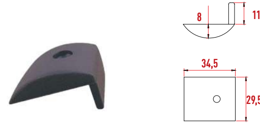
D124 Baza Denge Takoğu 8 mm
