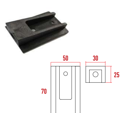
P1105-5 Gizli Ayak Bağlantı Pls. Kulaklı
