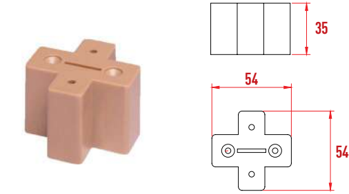
P3075 Mentese Yükseltici 35 mm
