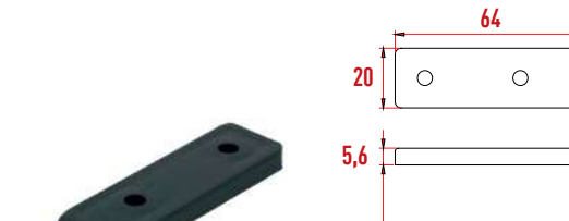
P3098 Alt Ara Bağlantı Plastiği
