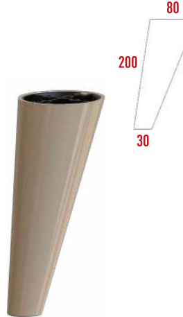
V318 Dupont Ayak 200 mm
