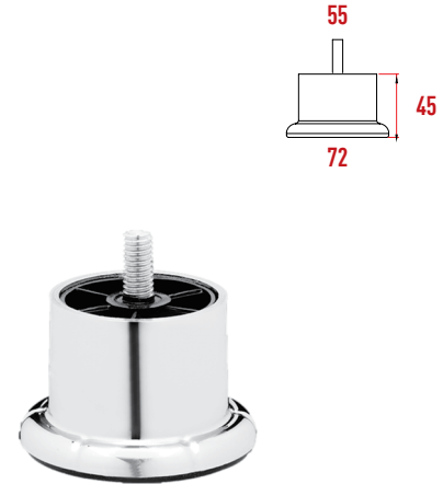
P980 Kelepir Ayak 45 mm
