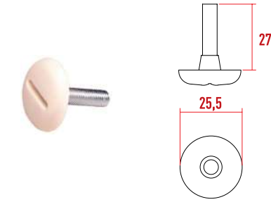
P1512 M6 Konik Bağlantı Vidası
