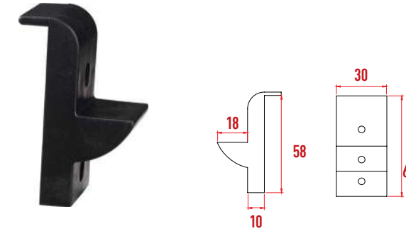
D303 Baza Stop Denge Plastiği
