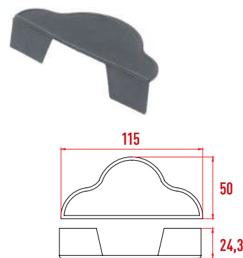
P1203 Üst Köşe Koruyucu
