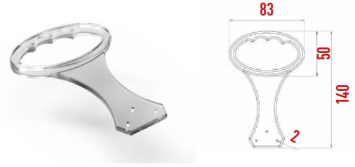
Y915 Plastik Baza Kulbu
