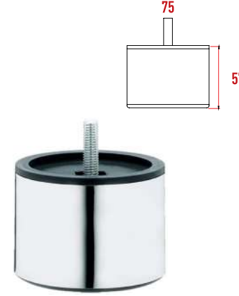
P1011 Luna Ayak 57 mm
