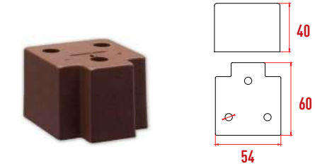
P3097 Plaza Mentese Yükseltici
