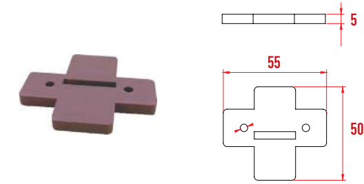
P3064 Mentese Yükseltici 5 mm
