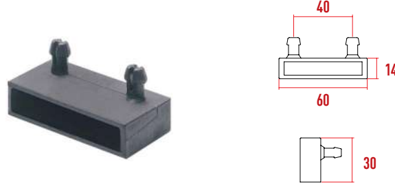
D124 Baza Denge Takoğu 8 mm
