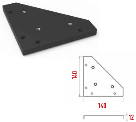
Y876 Üçgen Köşebent Üç Somunlu
