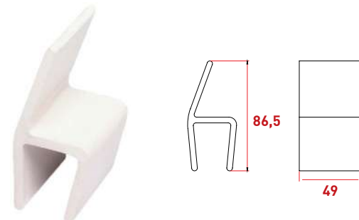
P2027 H Maşa
