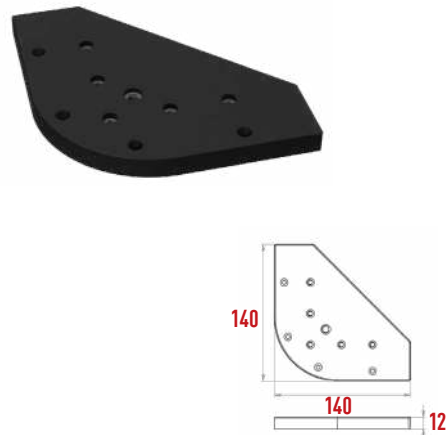
Y876 Üçgen Köşebent Üç Somunlu
