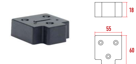
P3111 Enjoy Mentese Yükseltici 18 mm
