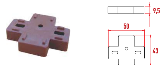
P3069 Mentese Yükseltici 9,5 mm
