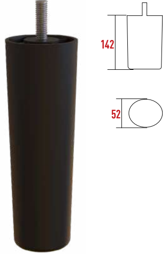
Y837 Gizli Ayak 142 mm
