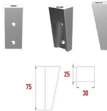
P1105-5 Gizli Ayak Bağlantı Pls. Çakmalı
