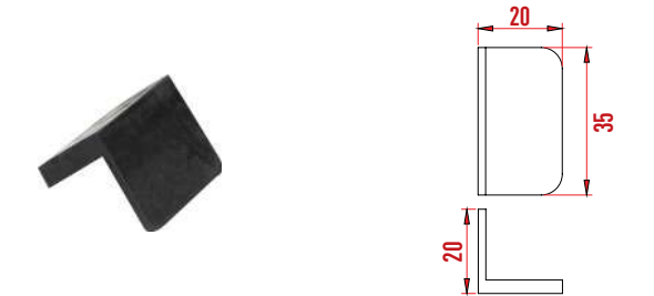
P1305-2 Boytaş Pvc L Siyah
