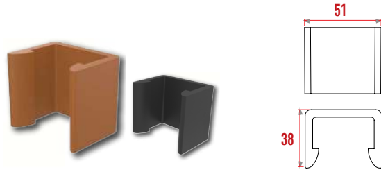
R279 Baza Birleştirici 40'lık
