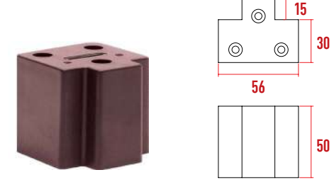
P3066 Kitaplık Ray Yükselticisi 50 mm
